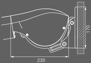
Top fix
